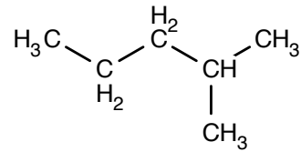
2-Methylpentaan
