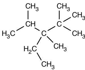
3-Ethyl-2,2,3,4-tetramethylpentaan
