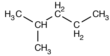
2-Methylpentaan
