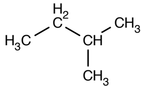
Pentaaan
