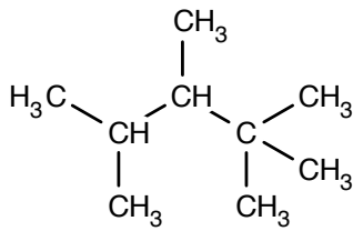
2,2,3,4-Tetramethylpentaan
