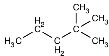
2,2-Dimethylpentaan
