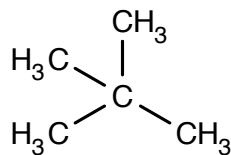
Dimethylpropaan
