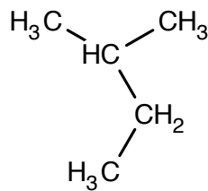
Methylbutaan
