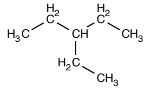
Ethylpentaan
