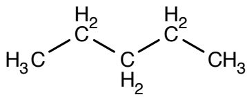
Pentaaan
