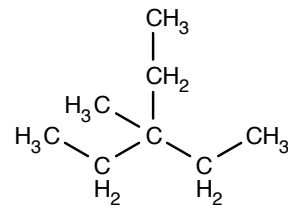
3-Ethyl-3-methylpentaan
